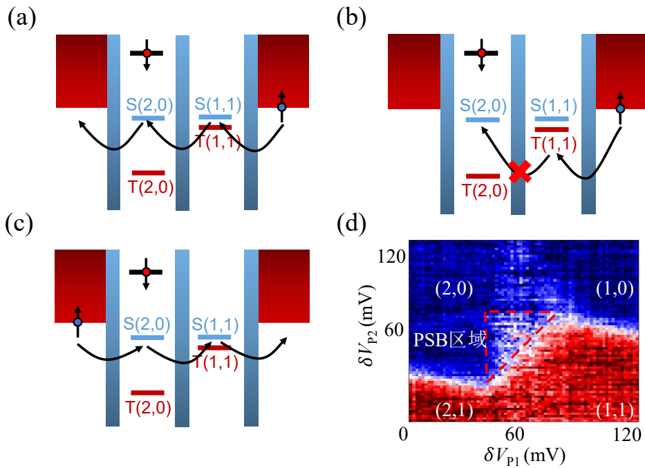
图 5.5 (a-c) 不同点间失谐情况下, 单重态 S 与三重态 T 的隧穿情况, a-b 图中在失谐小于 E_{ST} , 若形成的是 S(1, 1) , 空穴可以在双点之间自由隧穿, 若形成的是 T(1, 1) , 空穴的隧穿被阻塞。c 图中在失谐大于 E_{ST} , 即使形成原本被阻塞的三重态 T , 空穴也能够发生隧穿。(d) (1, 1)-(2, 0) 区域的泡利自旋阻塞区域, 图中使用红色虚线围起的三角形区域为泡利自旋阻塞区。
